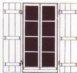
Fenêtre traditionnelle en bois : 0,80 x 1,60 m
